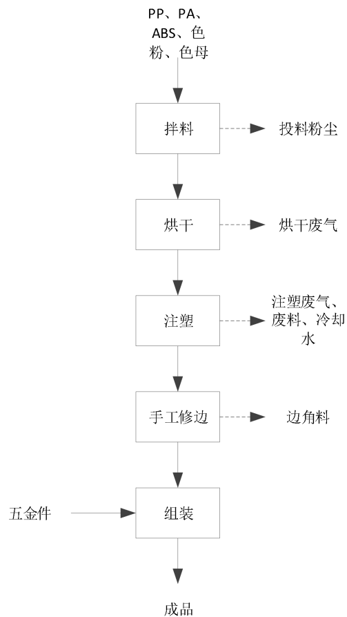
图 2-6 生产工艺及产污环节示意图（噪声伴随整个生产过程）
