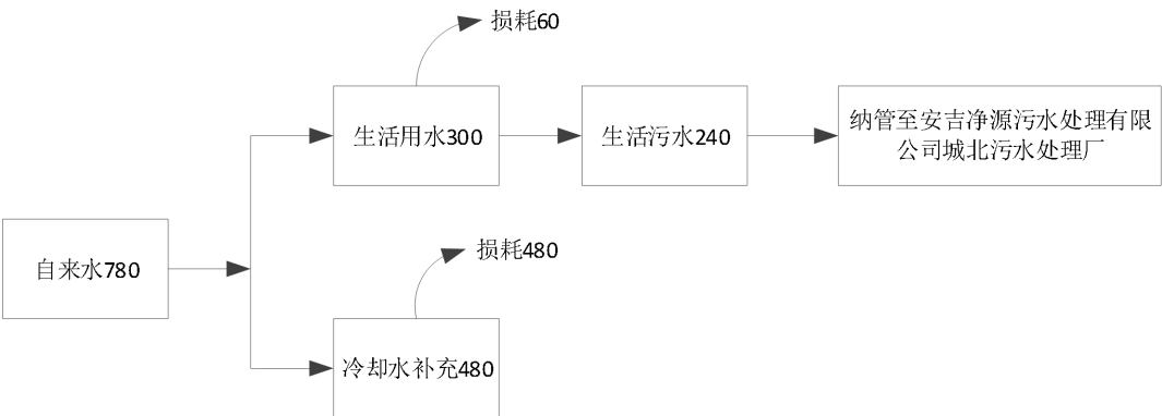
图 2-5 本项目营运过程水平衡图 (单位: t/a)
